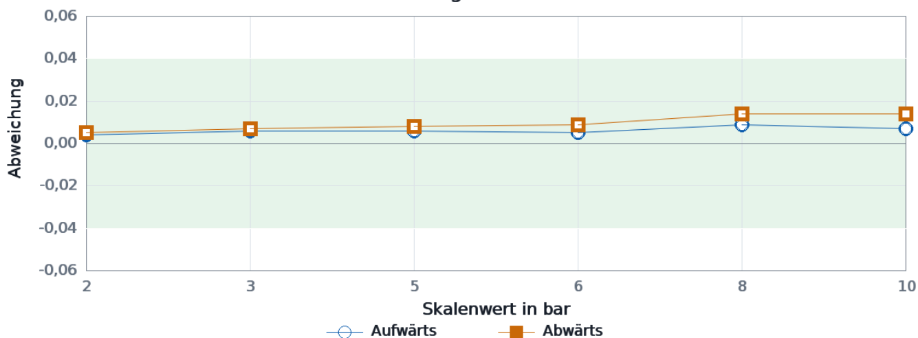
Abweichungskurve in bar
